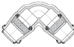
Tilausnro 6400 ISO pistoliitin PE-putkelle, kulma 90°
